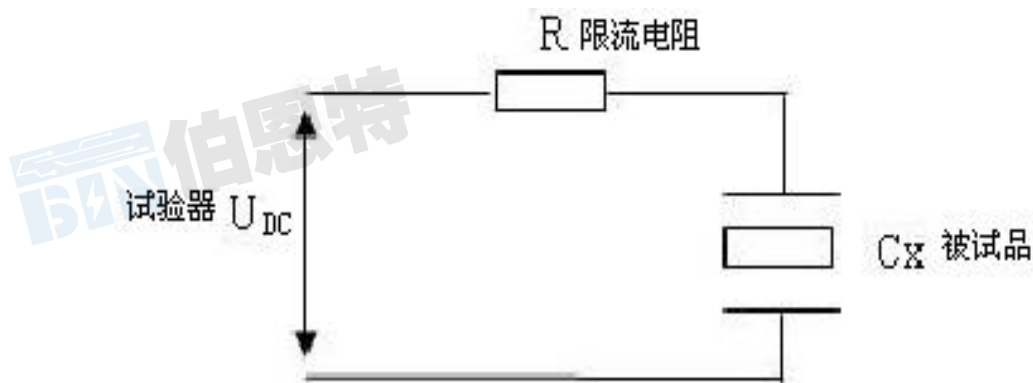
限流电阻使用示意图
