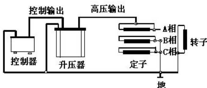
图 9 测量定子的某相连线图
