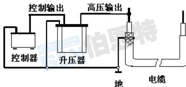
图 8 单相测量连线图
