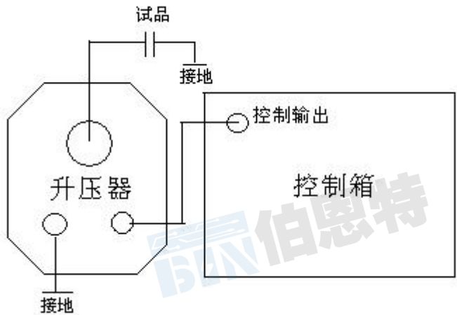
图 3 （连线图）
