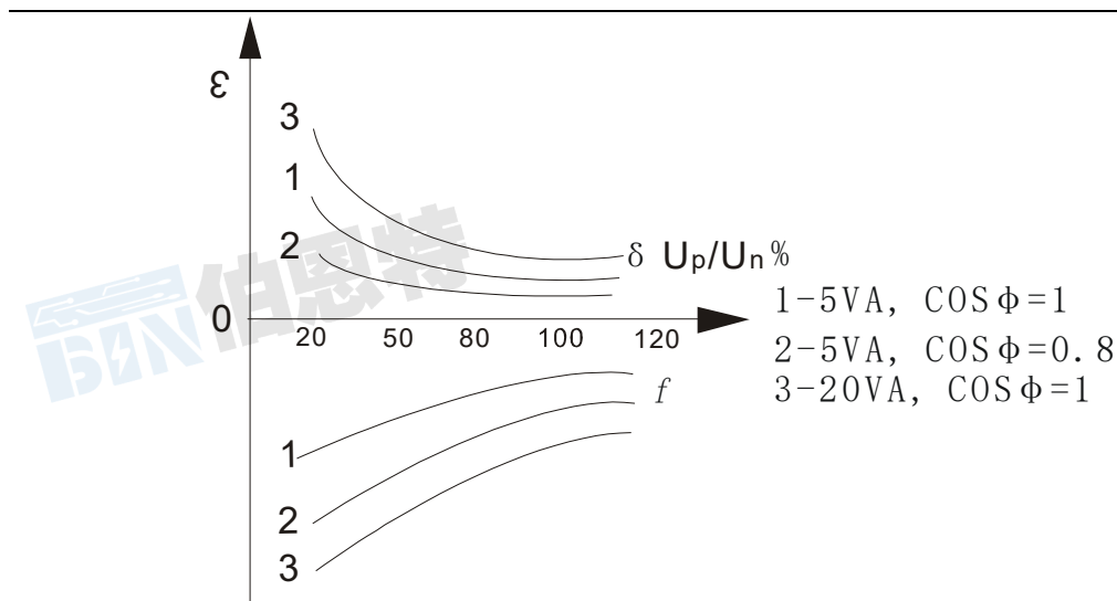
电压互感器电压与负荷特性
