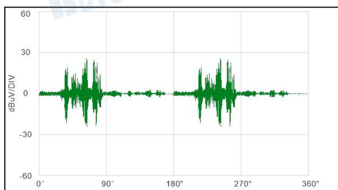
时域信号
