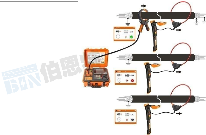
图 6- 18 带电识别(耦合法)接线检测
