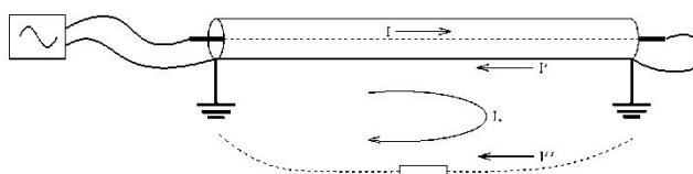
图 5-10 相线-护层接法信号流向示意图
