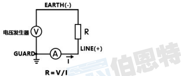
图 7- 6 绝缘电阻测量等效电路
