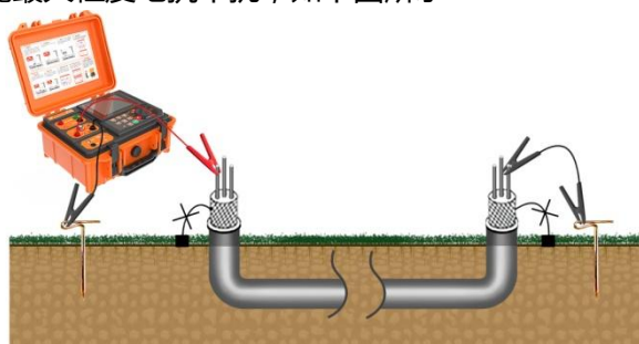
图 5-5 芯线-大地接法接线图
