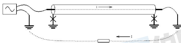
图 5-6 芯线-大地接法信号流向示意图
