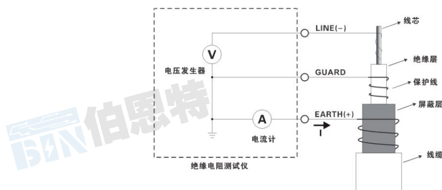
图 7-9 屏蔽端 GUARD 线使用示意图
